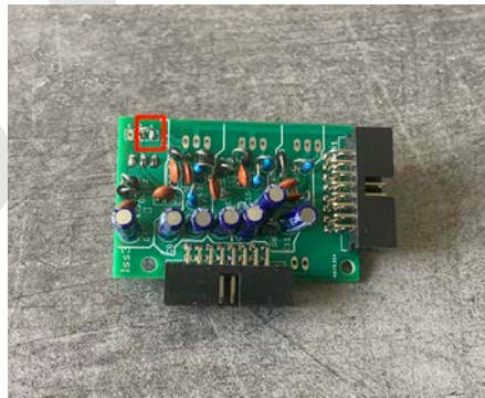
Implantation verticale des diodes.
